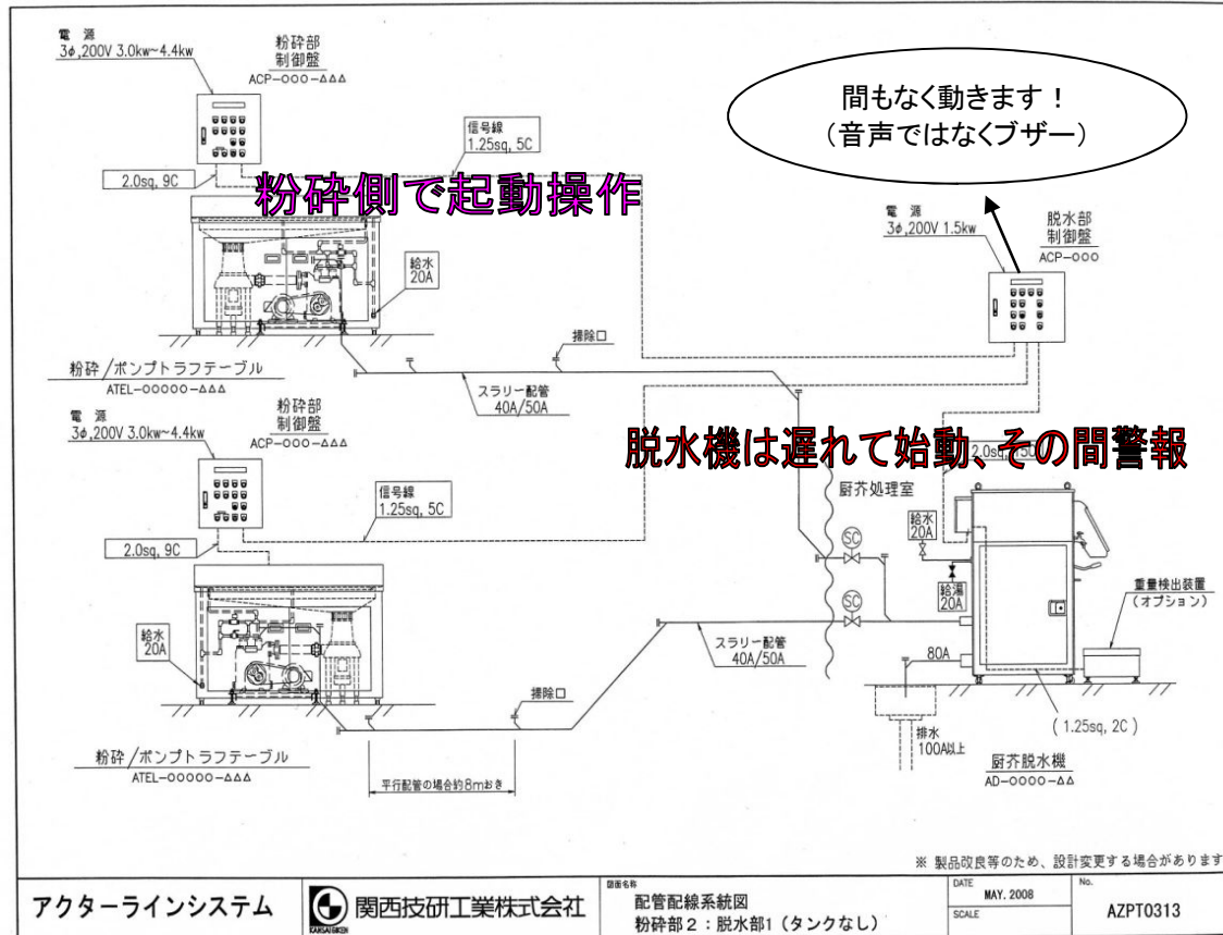
脱水機遅延運転・警報システム
